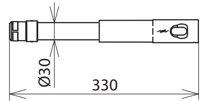
Maßbild AK 36 SK STK 330
