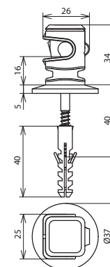
Maßbild LH DS 8 H16 HS5X50 KD8 GR
