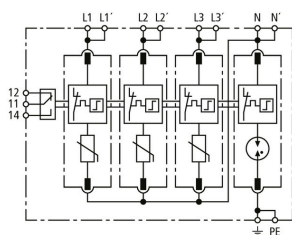
Prinzipialschaltbild DG MP TT 275 FM
