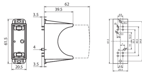
Maßbild DG PCB PV SCI 600
