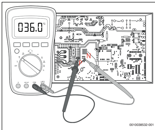
Bild 75 Spannung zwischen P und N
