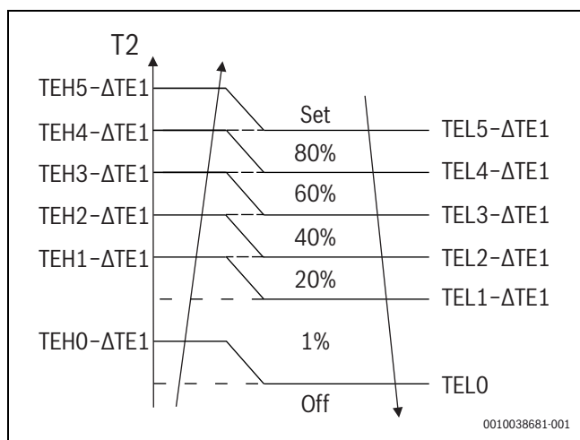
Bild 12 Anti-Kaltluft-Funktion
