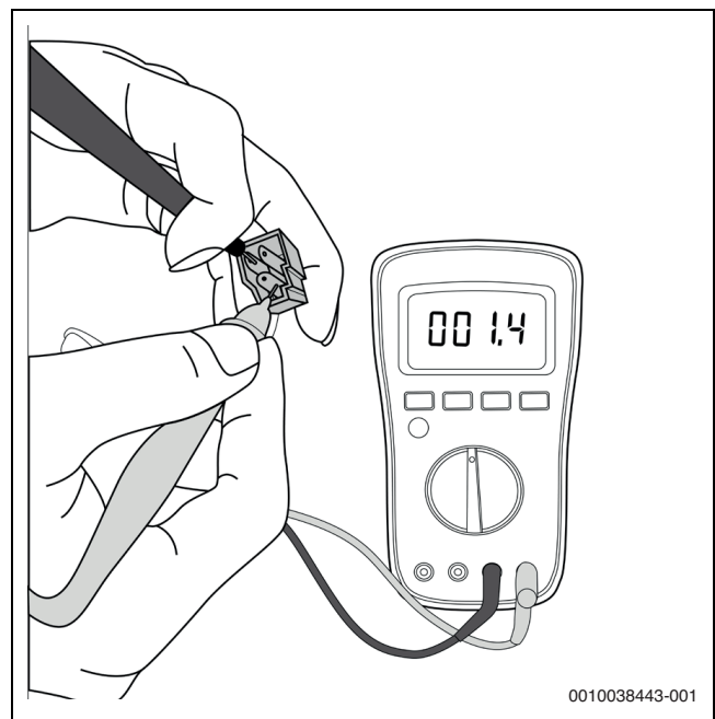
Bild 78 Kompressorprüfung
