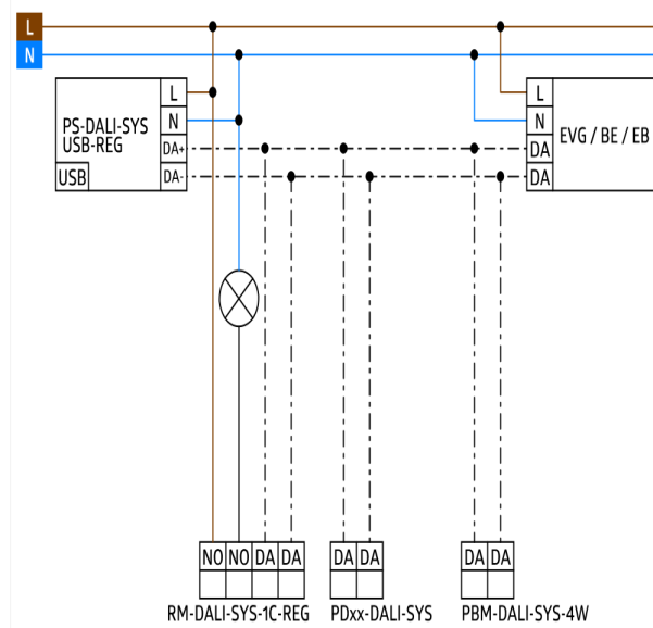
Schaltbild
