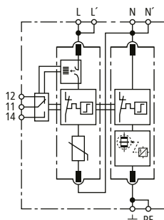
Prinzipialschaltbild
