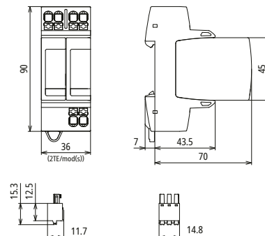
Maßbild
