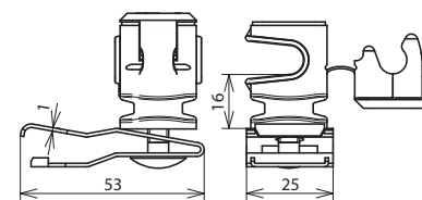
Maßbild LH FS 8 H16 K BR V2A
