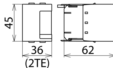
Maßbild DSE MOD 220
