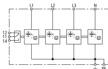
Prinzipschaltbild DSH B TNS 255 FM
