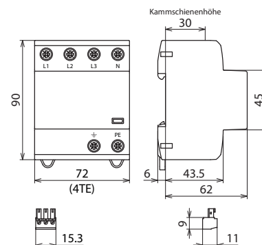
Maßbild DSH B TNS 255 FM
