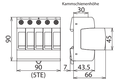
Maßbild DG M PV2 SCI 1000
