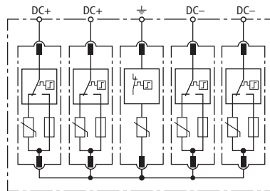
Prinzipialschaltbild DG M PV2 SCI 1000
