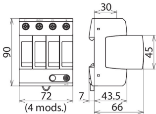
Maßbild DG MU 3PH 480 4W+G
