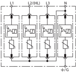
Prinzipialschaltbild DG MU 3PH 480 4W+G
