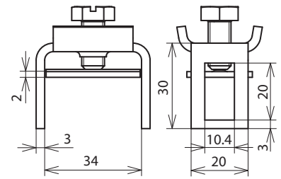
Maßbild RK FL30 PAS
