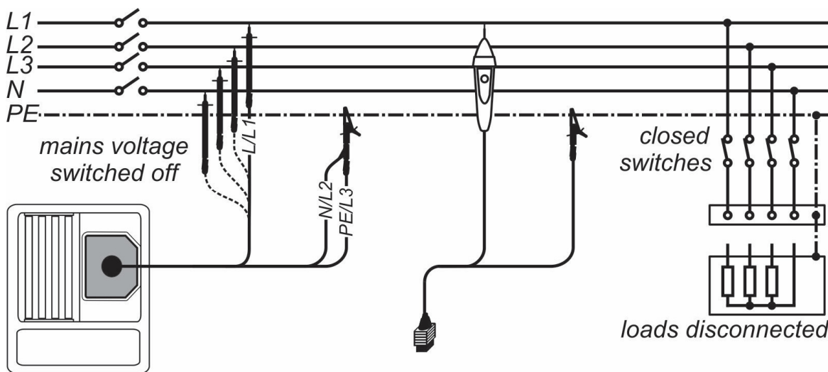
Afbeelding 5.6: Aansluiting van 3-geleider testdraad en de optionele Commander-testpen (044155)
