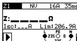
Afbeelding 5.26: Leidingsimpedantie
