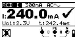
Afbeelding 5.20: Voorbeeld activeringsstroommeting
