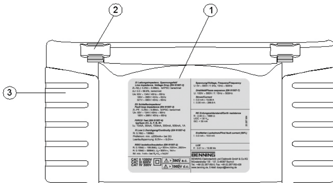
Afbeelding 3.5: Onderaanzicht
