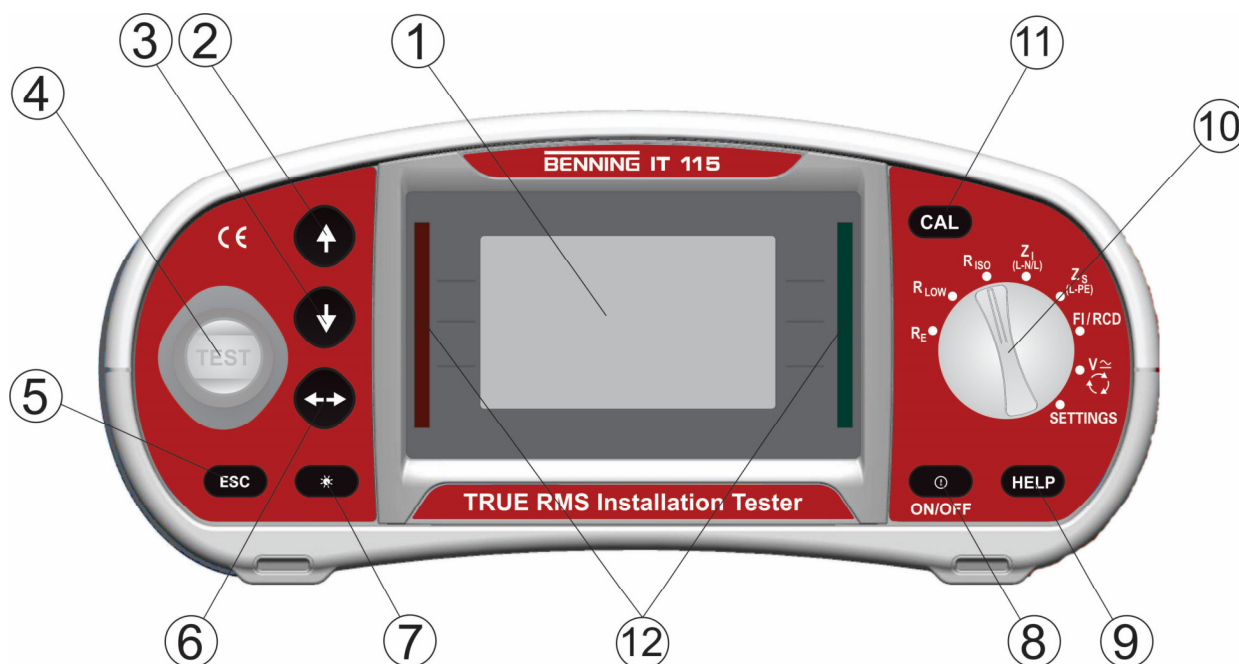
Afbeelding 3.1: Voorzijde
