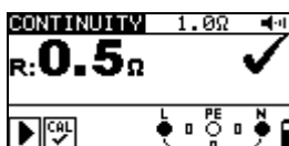
Afbeelding 5.12: Voorbeeld doorgangsmeting
