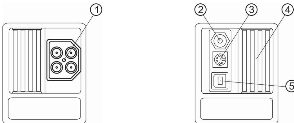
Afbeelding 3.2: Aansluitpaneel
