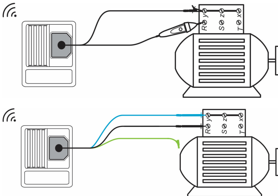
Afbeelding 5.11: Gebruik van de optionele Commander-testpen (044155) en 3-geleider testdraad
