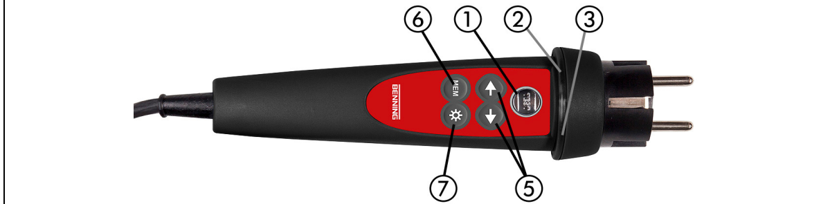
Afbeelding C.2: Voorzijde van Commander-teststekker voor stopcontact met randaarde (schakelbaar met TEST-toets) (044149)
