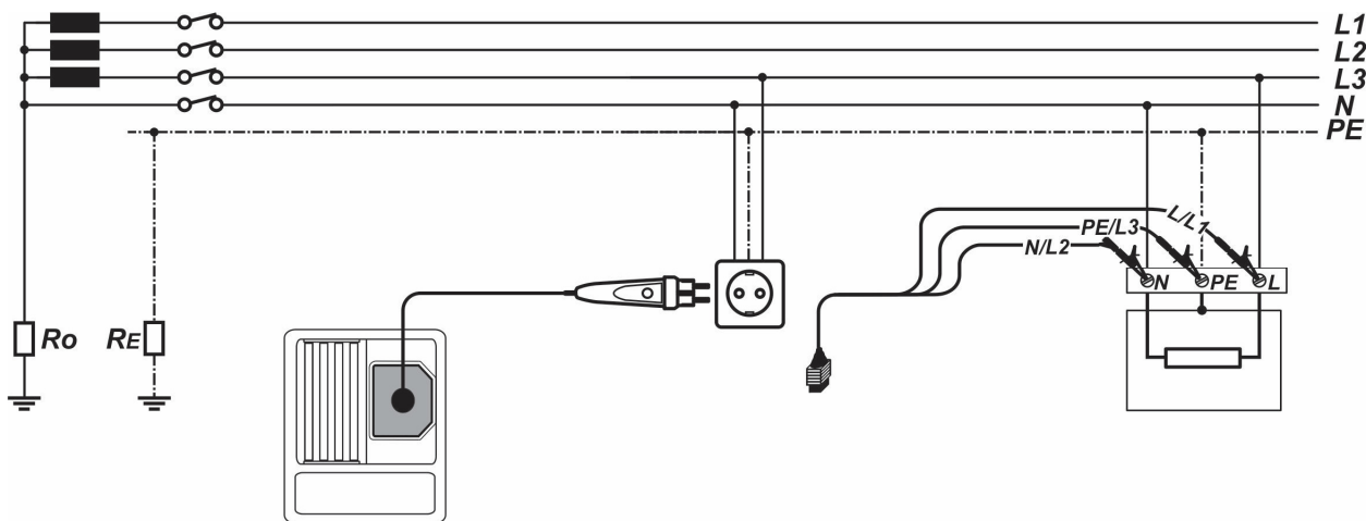
Afbeelding 5.24: Aansluiting van de optionele Commander-teststekker (044149) en van de 3-geleider testdraad
