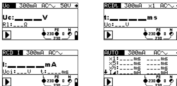
Afbeelding 5.16: RCD-controles
