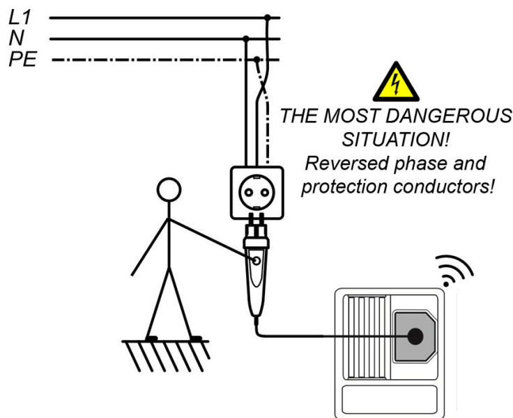
Afbeelding 5.36: Omgewisselde L- en PE-geleider – fasespanning op PE-geleider wordt herkend door de TEST-toets op de Commander-teststekker (optie) aan te raken.
