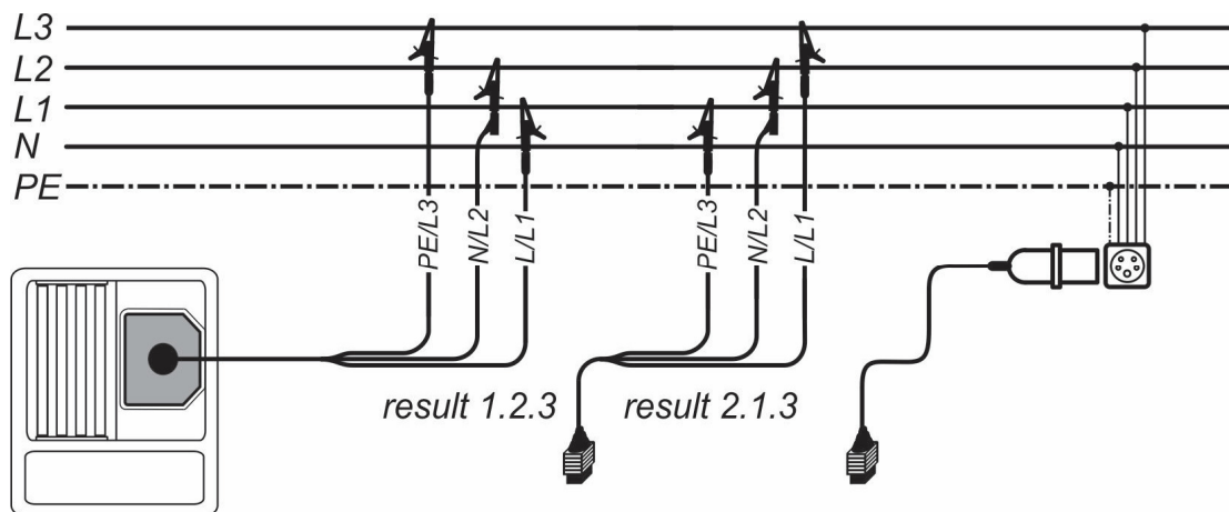
Afbeelding 5.2: Aansluiting van 3-geleider testdraad en optionele CEE-meetadapter (044148) in driefasesysteem
