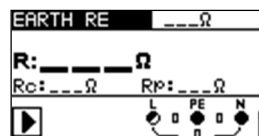
Afbeelding 5.32: Aardingsweerstand
