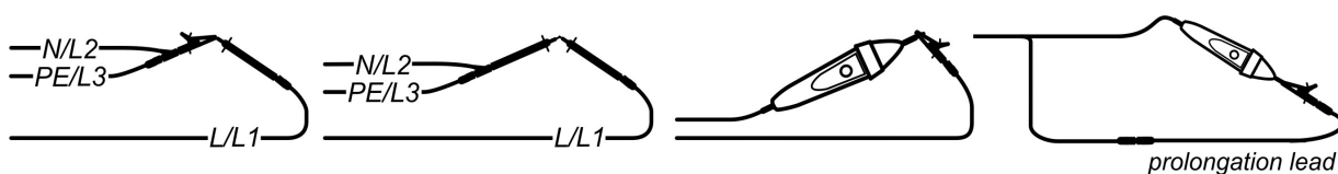
Afbeelding 5.13: Kortgesloten 3-geleider testdraad en de optionele Commander-testpen (044155)
