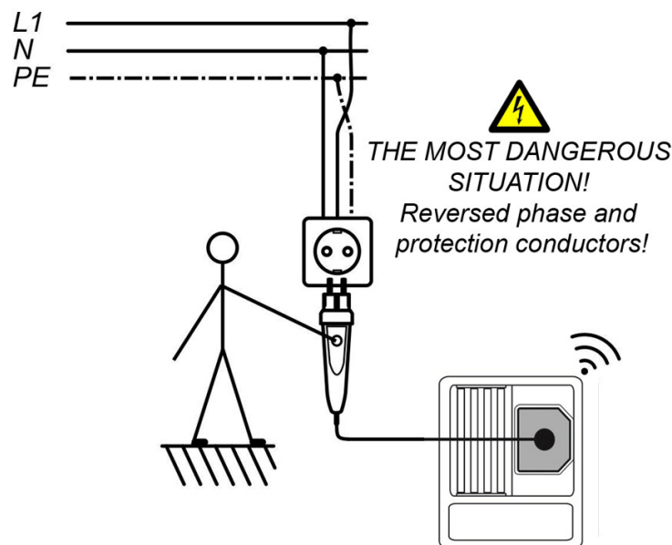
Afbeelding C.4: Verwisselde L- en PE-geleider – fasespanning op PE-aansluiting wordt herkend door de TEST-toets op de optionele Commander-teststekker (044149) aan te raken.
