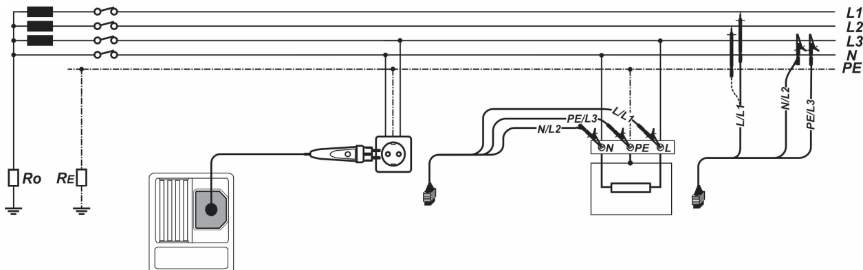
Afbeelding 5.28: Aansluiting van de optionele Commander-teststekker (044149) en van de 3-geleider testdraad
