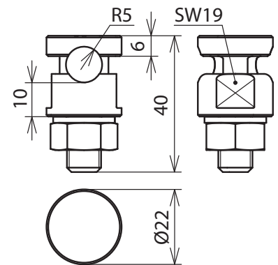
Maßbild KSV 200 10 FER V2A
