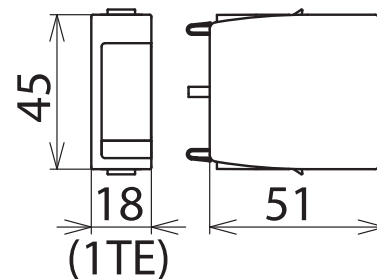
Maßbild DG MOD 275
