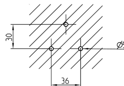
Bohrbild
