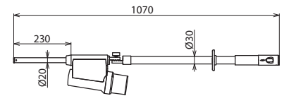
Maßbild PHE4 10 S ZK
