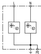
Prinzipialschaltbild DSH TN 255
