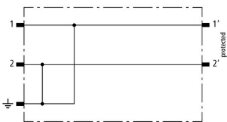
Prinzipschaltbild BCO M2 E
