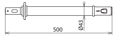
Maßbild H STK 43 500
