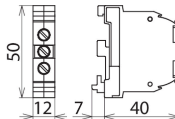
Maßbild SLK 16
