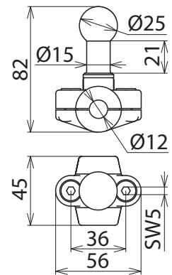
Maßbild KFP 25 RL 12
