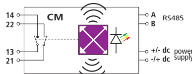
Principalschaltbild DRC MCM AL XT
