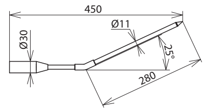
Maßbild PSO M8 W25 PHE
