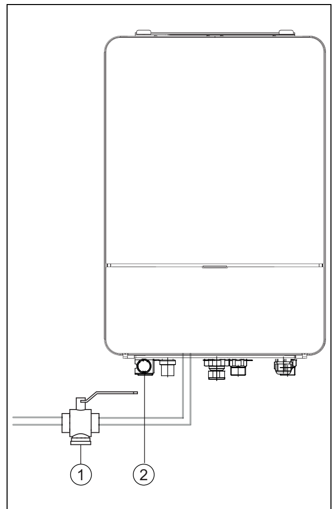
Bild 7 Inneneinheit AWB
