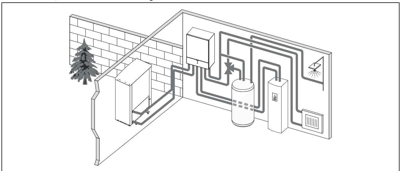
Bild 3 Wärmepumpe Compress 7000i AW, Inneneinheit AWB ohne elektrischen Zuheizler, externer Warmwasserspeicher und externer Zuheizler
