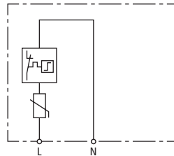
Prinzipschaltbild
