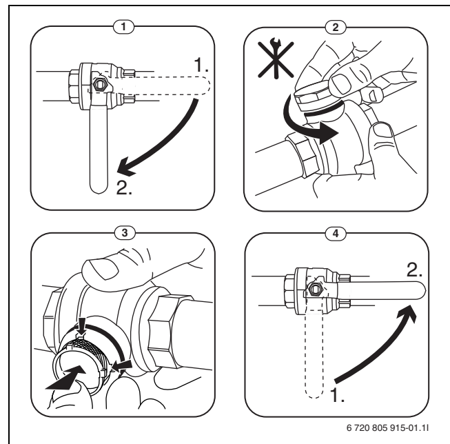
Bild 8 Siebreinigung
