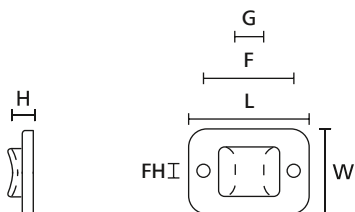
TY3G1 (Seitenansicht)
