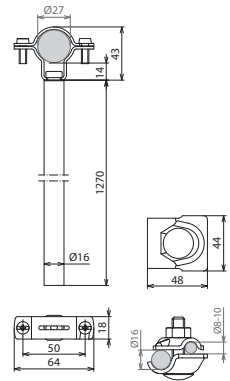
Maßbild DIDH PAE 27 D16 1270 AL V2A
