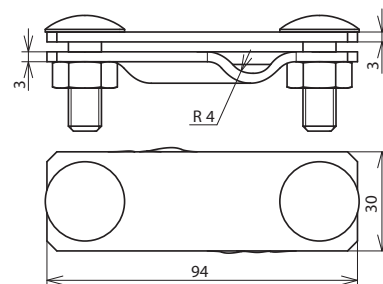
Maßbild SVK 7.10 FL30 V4A
