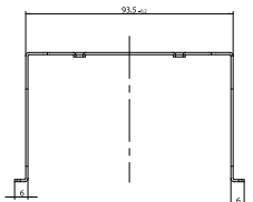
Vorderansicht AH96 für das UMG 96RM
