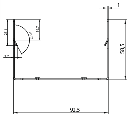
Vorderansicht AH96 für das UMG 96L / UMG 96
