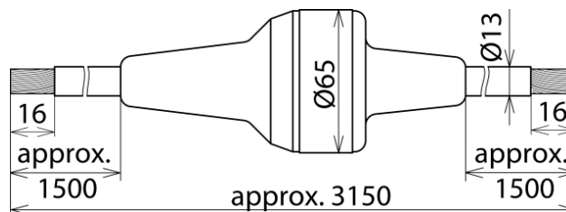
Maßbild EXFS KU
