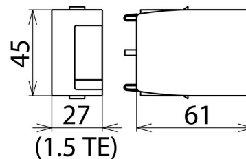
Maßbild DG MOD E H LI 1000
