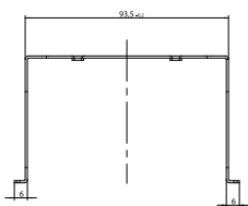
Vorderansicht AH96 für das UMG 96RM
