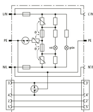
Prinzipschaltbild DPRO 230 NT
