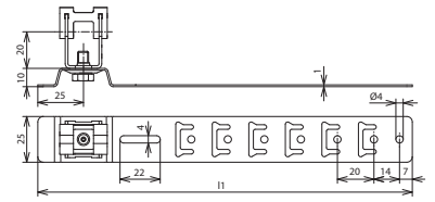
Maßbild DLH UG 8 H20 L205 V2A
