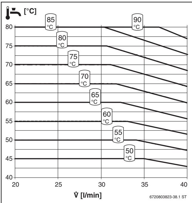
Bild 60 Temperaturverhalten Einzelstation FF40S
