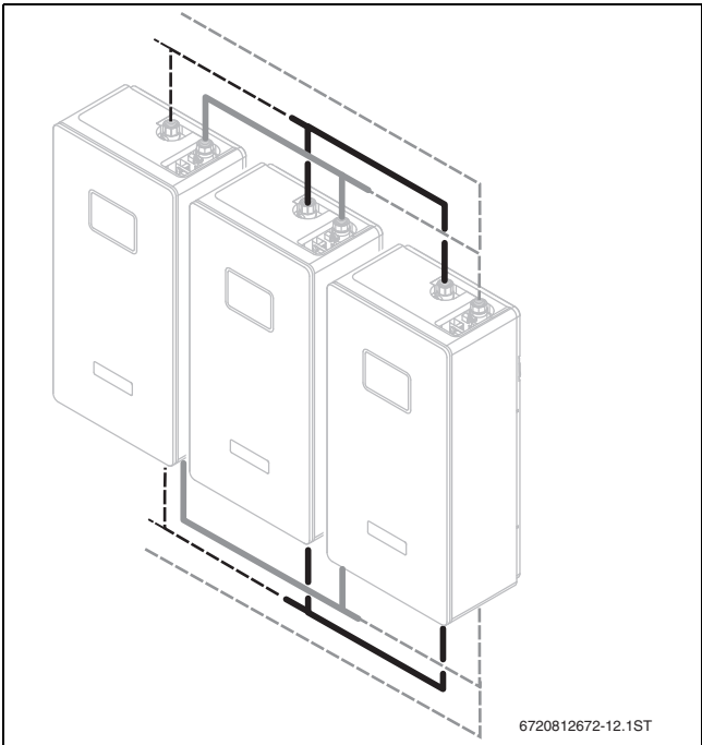
Bild 27 Beispiel: FF120S mit Verrohrungssatz (Tichelmann-Prinzip)
