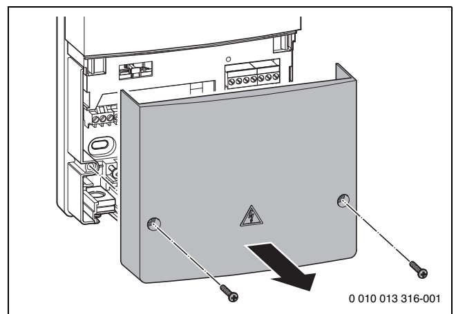
Bild 46 Modul öffnen
