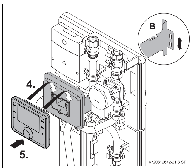
Bild 39 Bedieneinheit montieren
