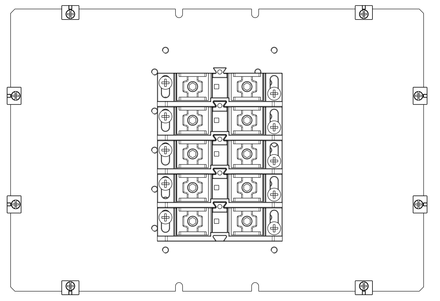
Abox-i 1500-150 2/5
