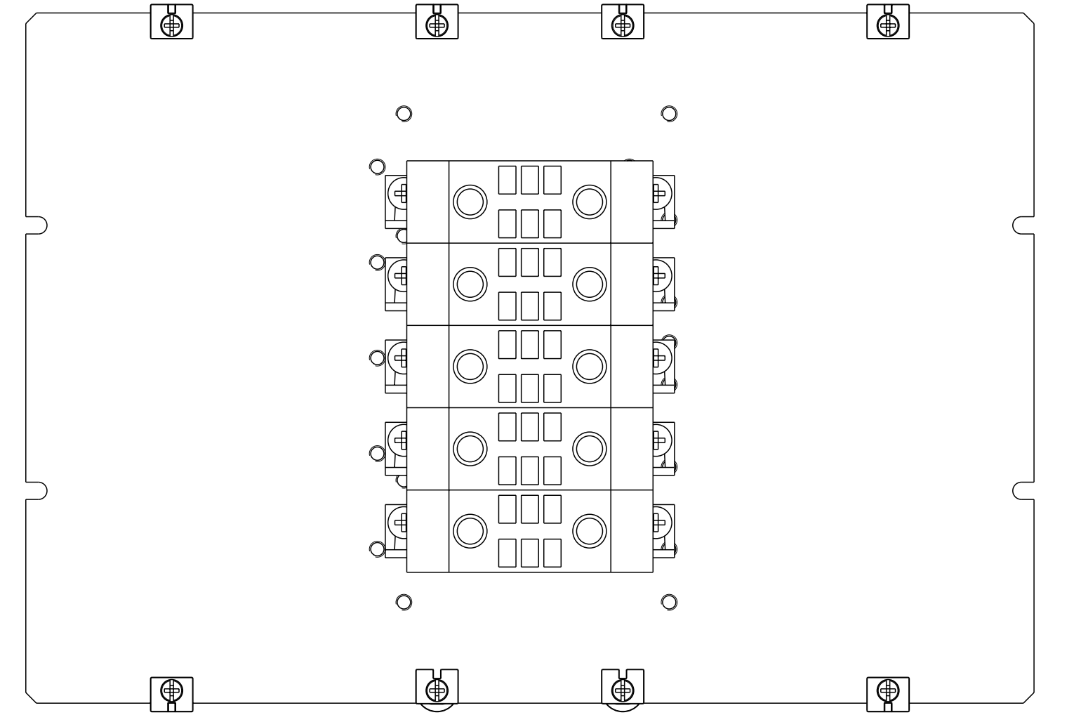
Abox-i 1500-DK-150 2/5
