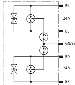
Prinzipschaltbild
