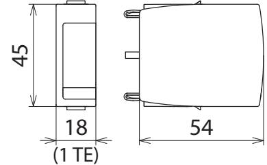
Maßbild
