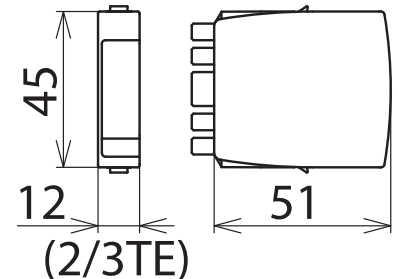
Maßbild BXT ML2 BD HFS 5
