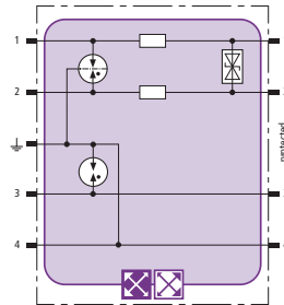
Prinzipschaltbild BXT ML2 BD HFS 5
