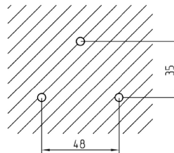
Bohrbild
