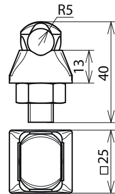
Maßbild KSV 6.10 CU
