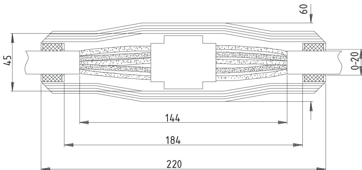
Klemmstein KS-0
