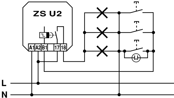
3-Leiter Anschluss
