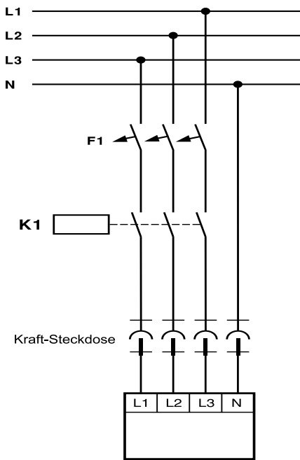
Elektroherd
