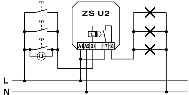
4-Leiter Anschluss
