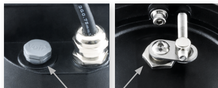
selbstentlüftendes Ventil
