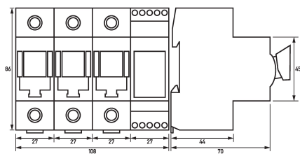
Maßzeichnung Gruppenansicht
