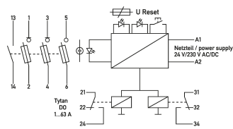
Anschlussschema
