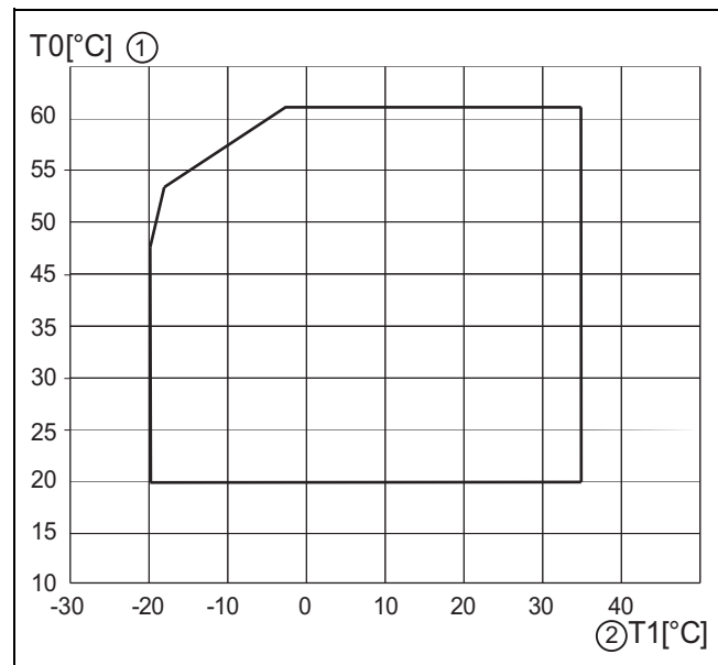
Bild 1 Wärmepumpe ohne Zuheizler
