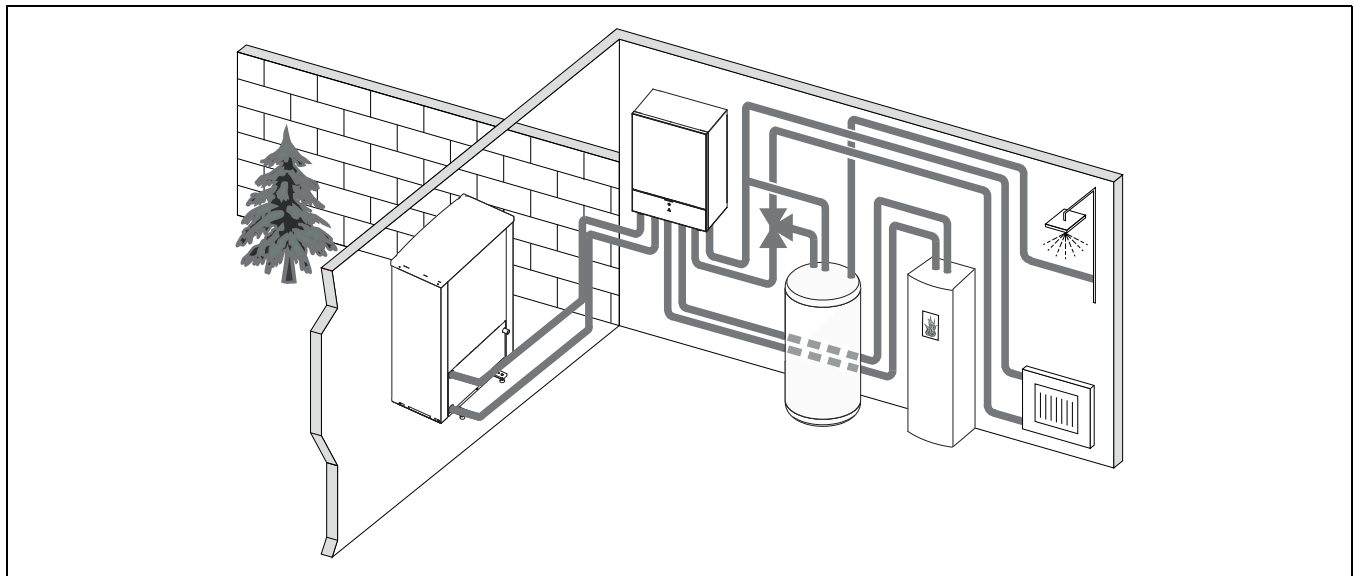
Bild 3 Wärmepumpe Compress 7001i AW, Inneneinheit AWB ohne elektrischen Zuheizter, externer Warmwasserspeicher und externer Zuheizter
