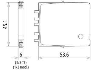
Maßbild BCO MOD ML2 EX 24
