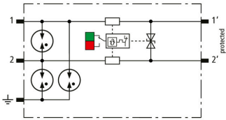
Prinzipialschaltbild BCO MOD ML2 EX 24
